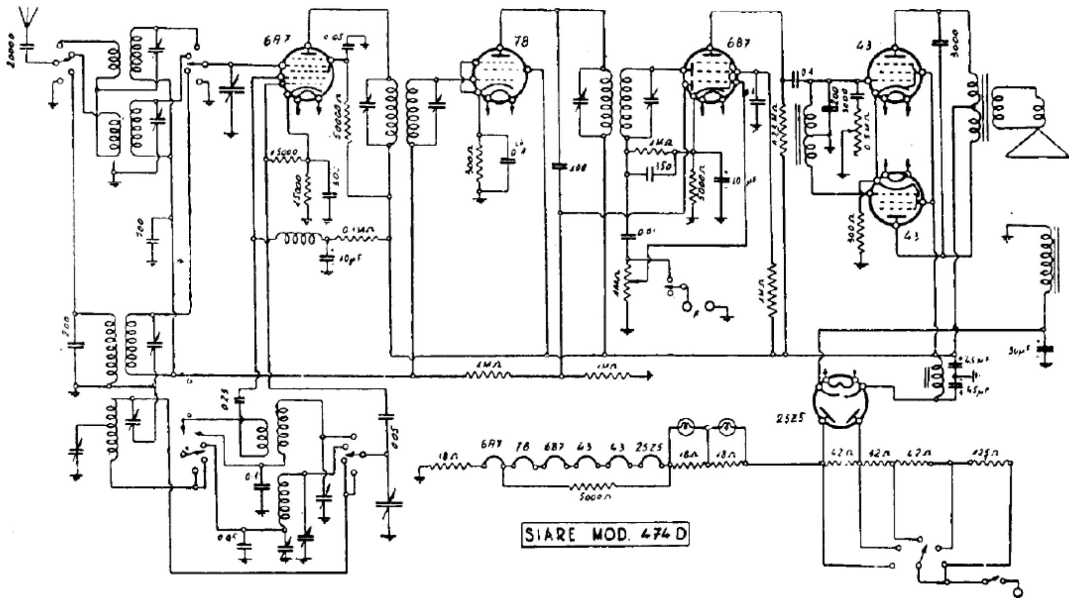
RADIO SIARE — Modello « 474 D ». • Produzione 1936. Media frequenza: 348 kc
